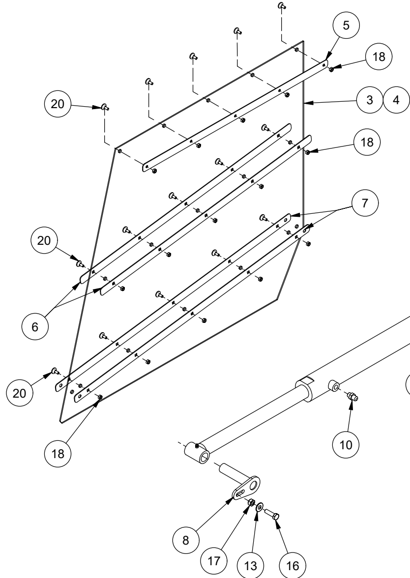
HYDRAULIC OFFSET DÉPORT HYDRAULIQUE
