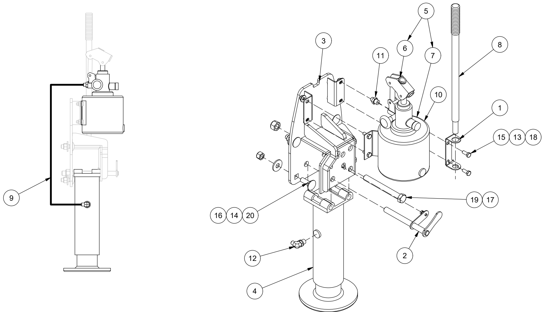
HYDRAULIC SCHEMA / SCHÉMA HYDRAULIQUE
