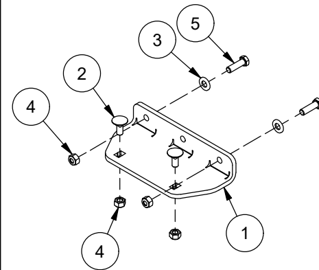
BELT MANUAL OFFSET DÉPORT MANUEL À COURROIE
