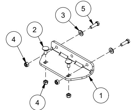
BELT MANUAL OFFSET DÉPORT MANUEL À COURROIE
